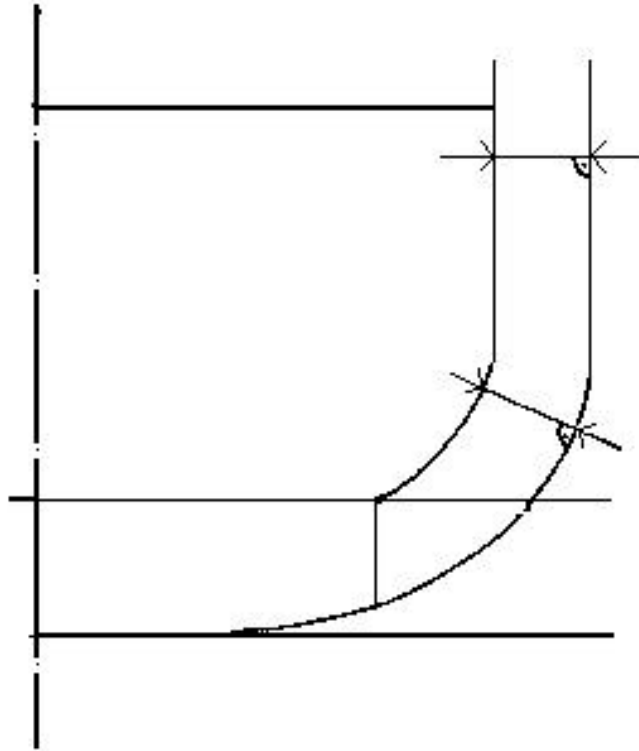
Figura 2: Definición de los límites de los tanques de carga a efectos del párrafo 4)
