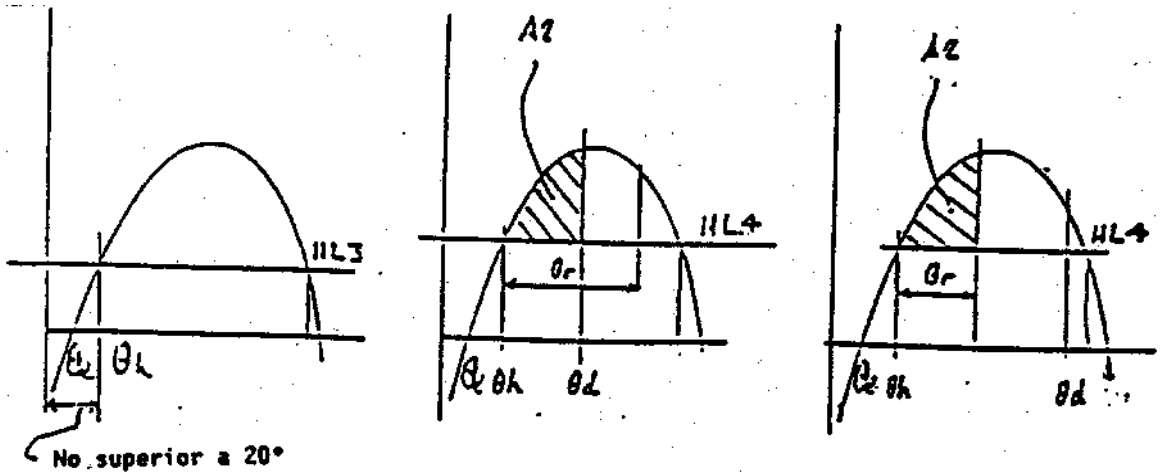
Figura 2 - Estabilidad con avería
